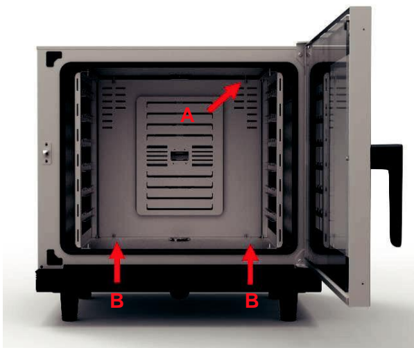
Rysunek 47. Śruby mocujące płytkę ssącą do BAKE PRO
